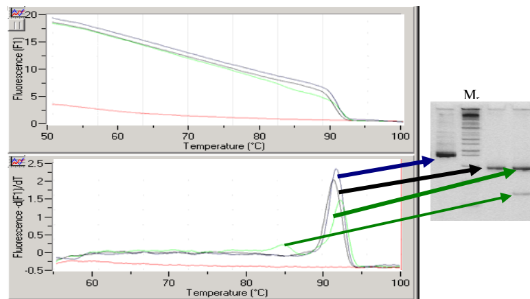
รูปที่ 4 แสดงการวัด fluorescence จาก PCR product เมื่อมีการเพิ่มอุณหภูมิขึ้นเรื่อยๆ ในกรอบบน และเมื่อเปลี่ยน scale ให้เป็น dF/dT จะได้กราฟดังรูปในกรอบล่าง ซึ่งแสดงอุณหภูมิที่เป็น melting temperature ของ PCR product แต่ละตัว โดยเทียบกับขนาดเมื่อ run gel electrophoresis ตามที่ลูกศรชี้
